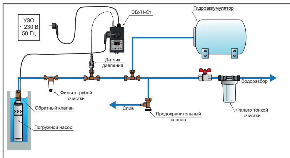
Пример 4. Подключение ЭБУН-Ст к погружному насосу.
