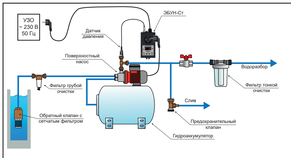
Пример 3. Подключение ЭБУН-Ст к поверхностному насосу или насосной станции.
